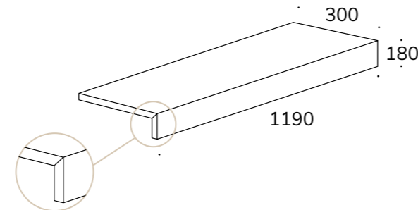
Vela 120
